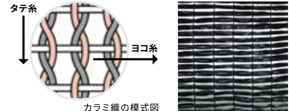
カラミ織の模式図
