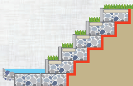
蛇籠・布団籠の吸出し防止
