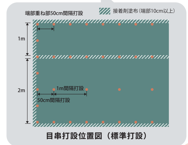
仮止めし、目串打設箇所にマーキングを行います
